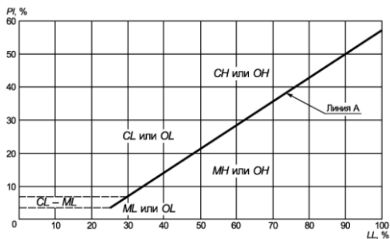
Рисунок Е.3 — График пластичности грунтов
